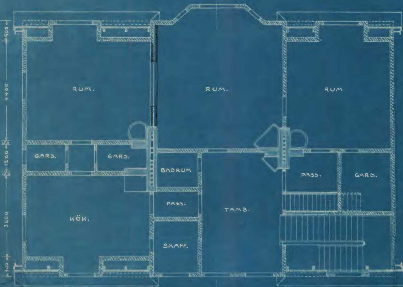
BOTTEN PLAN.
