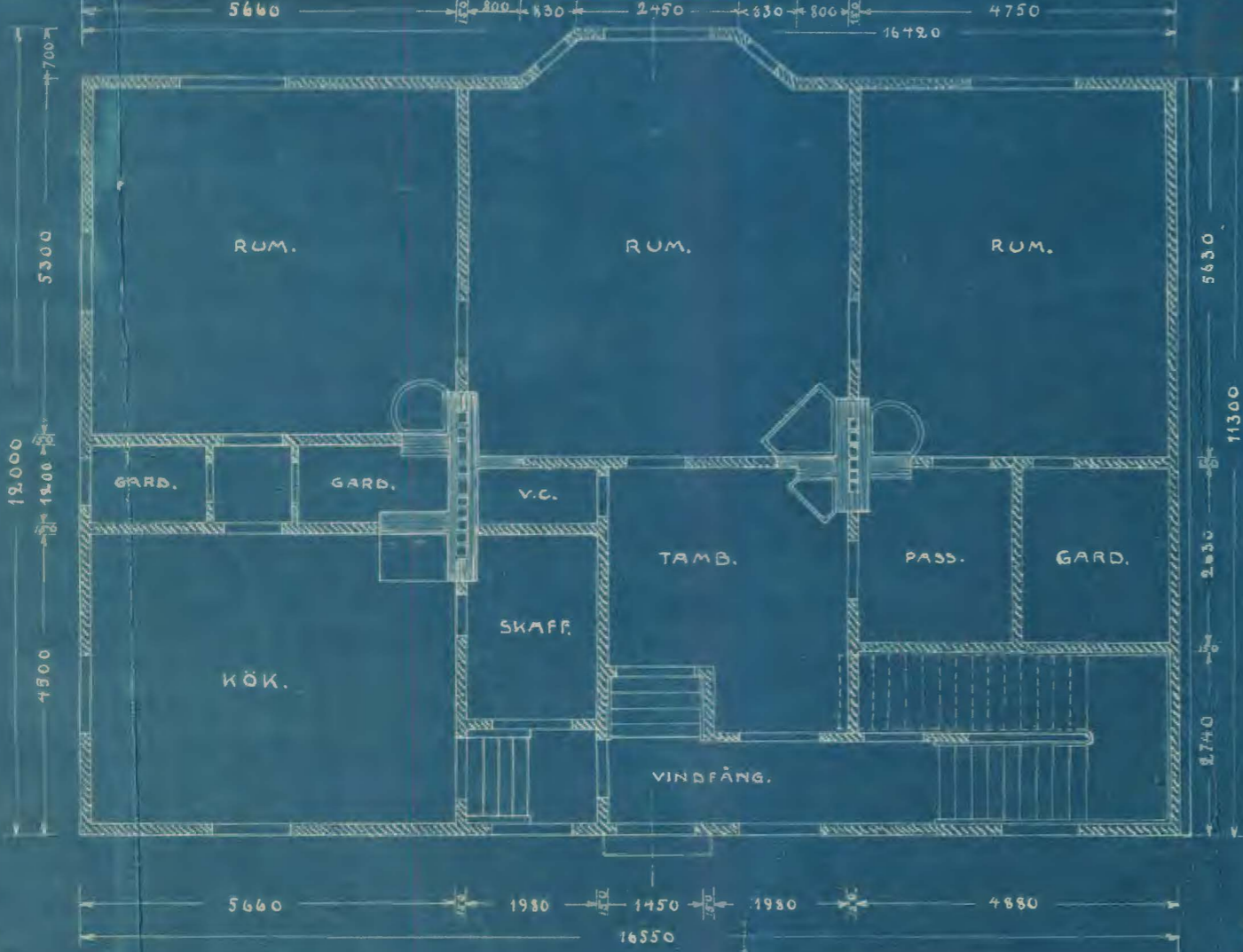
BOTTEN PLAN.
